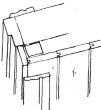
Näide horisontaallaudise sisenurga detailidest.
